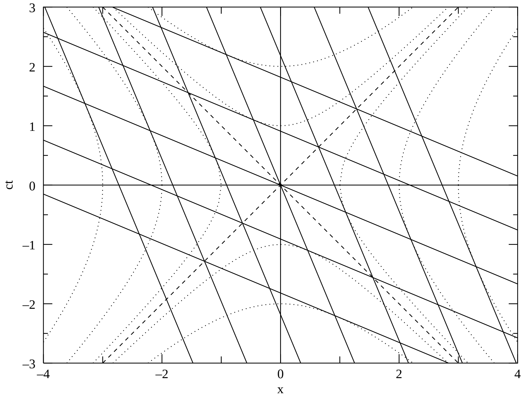
Minkowski Diagram–
